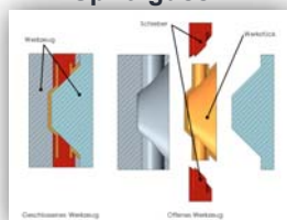
Spritzguss
