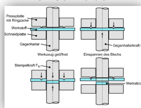
Feinschneiden
