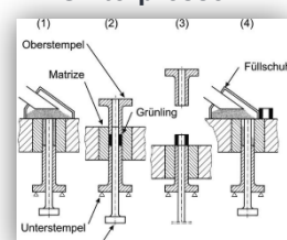
Sinterpressen
