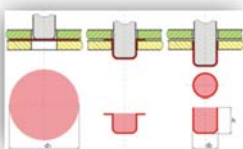
Tiefziehen
